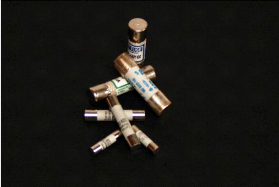
Sandfyldt finsikring 250mA, 6x32mm, 1000V
